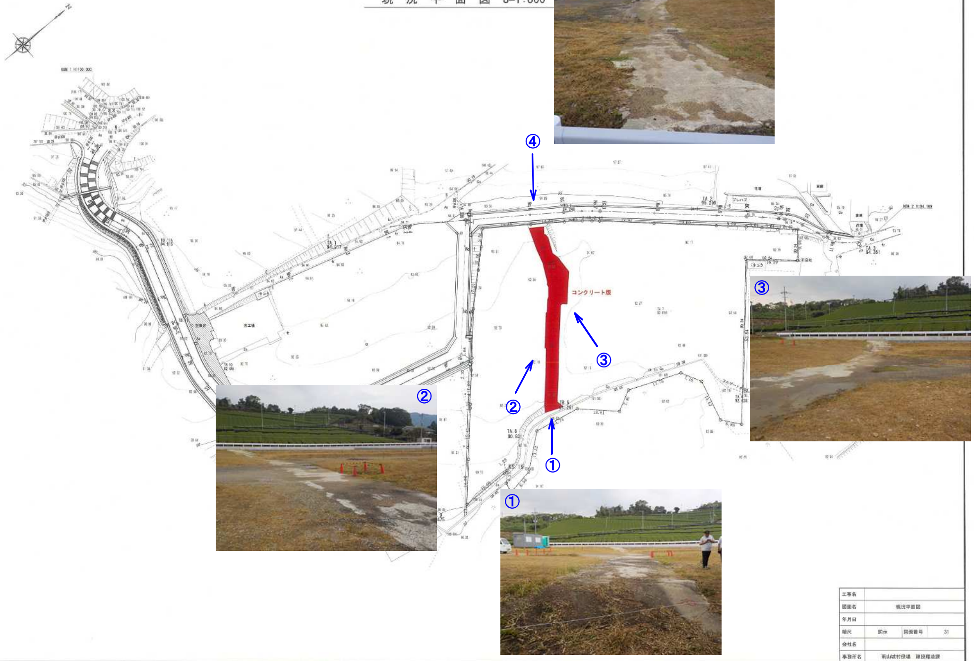
現況平面図 S=1:800
